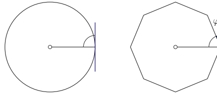
Abbildung 2.7: Beim Kreis steht der Radius senkrecht zur Kreislinie (links). Bei einem Polygon ist der Winkel zwischen Radius und Umfangslinie nicht ganz rechtwinklig (rechts).
